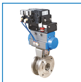
Pacchetto di automazione con valvola a sfera wafer, attuatore pneumatico e posizionale elettropneumatico. Automation package with wafer ball valve, pneumatic actuator and electropneumatic positioner.
